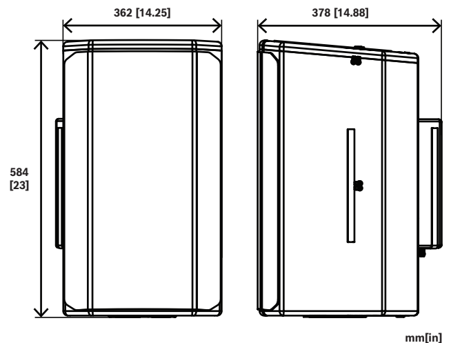
Fig. 1: Dimensions
