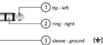
PHONES Jack stereo
