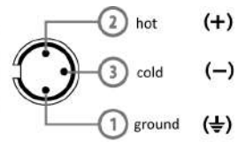
MIC INPUT XLR bilanciato maschio
