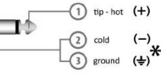
LINE IN, OUT vari Jack (sbilanciato)
