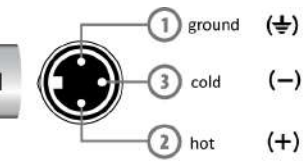
MAIN MIX OUT XLR bilanciato femmina
